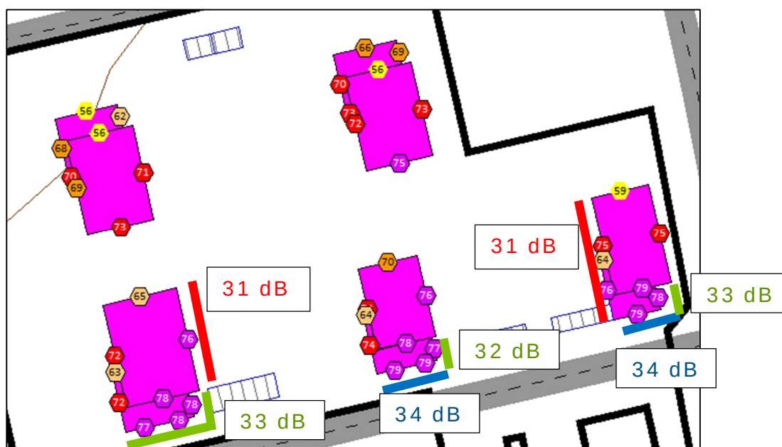
Kuva 21 Julkisivuille kohdistuvat ääneneristävyydsvaatimukset enimmäisäänitasojen LAF_{max} perusteella vaiheessa 1. niiltä osin, kun minimivaatimus 30 dB ylittyy.
